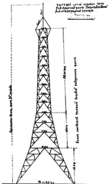
Антенные мачты Петропавловской радиостанции (ККОМ, НВФ 2536; 2728)
